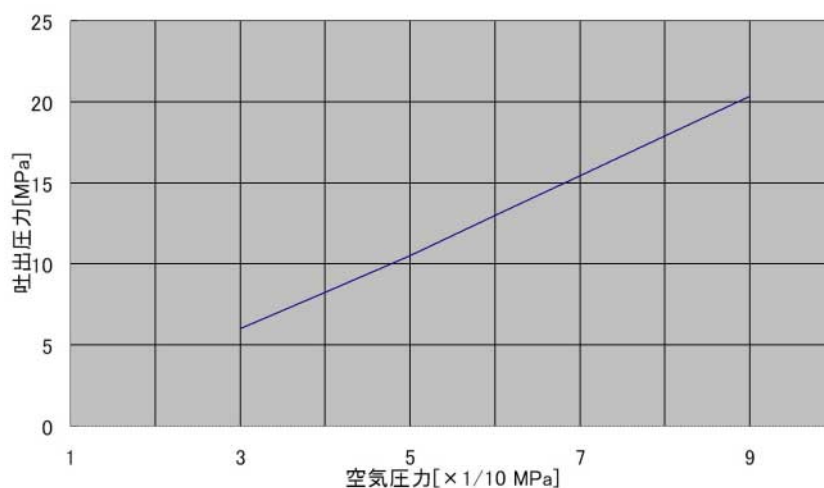
KSP-402性能曲線
